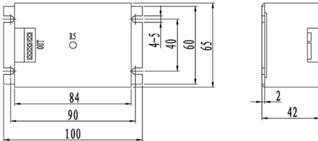
専用電源 LDD-800A(入力電圧 A C 100V)
