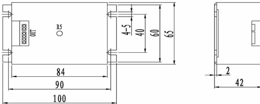
専用電源 LDD-800A 外観図
